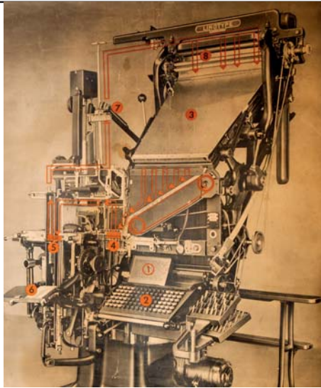
Linotype-Setzmaschine
